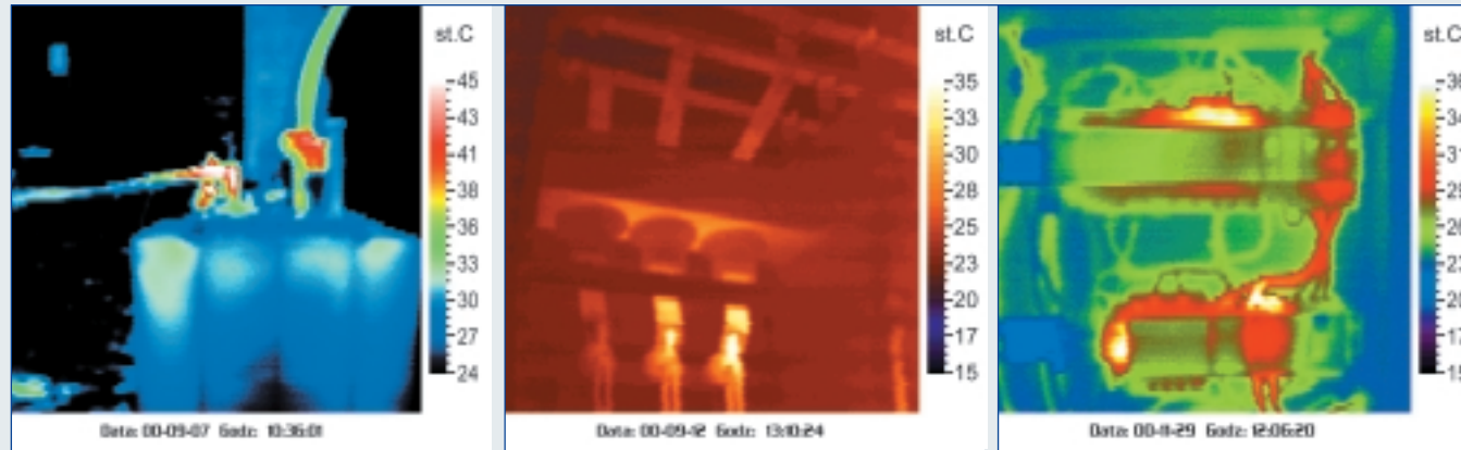
Transformator wysokiego napięcia Rozdzielnia napięcia 15kV Rozdzielnia 220V
