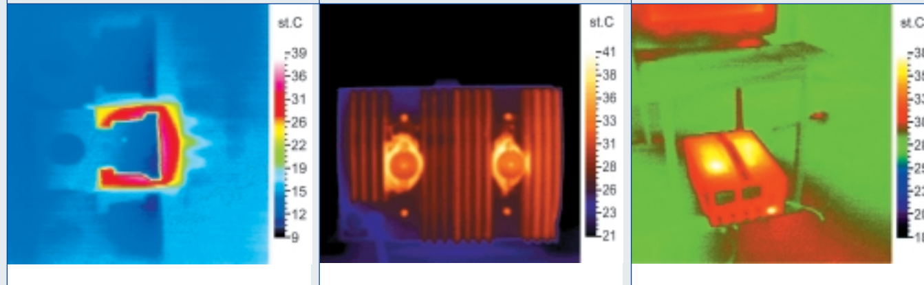
Stabilizator napięcia w obudowie T0220 Zasilacz laboratoryjny-radiator Zasilacz laboratoryjny. Widok z góry
