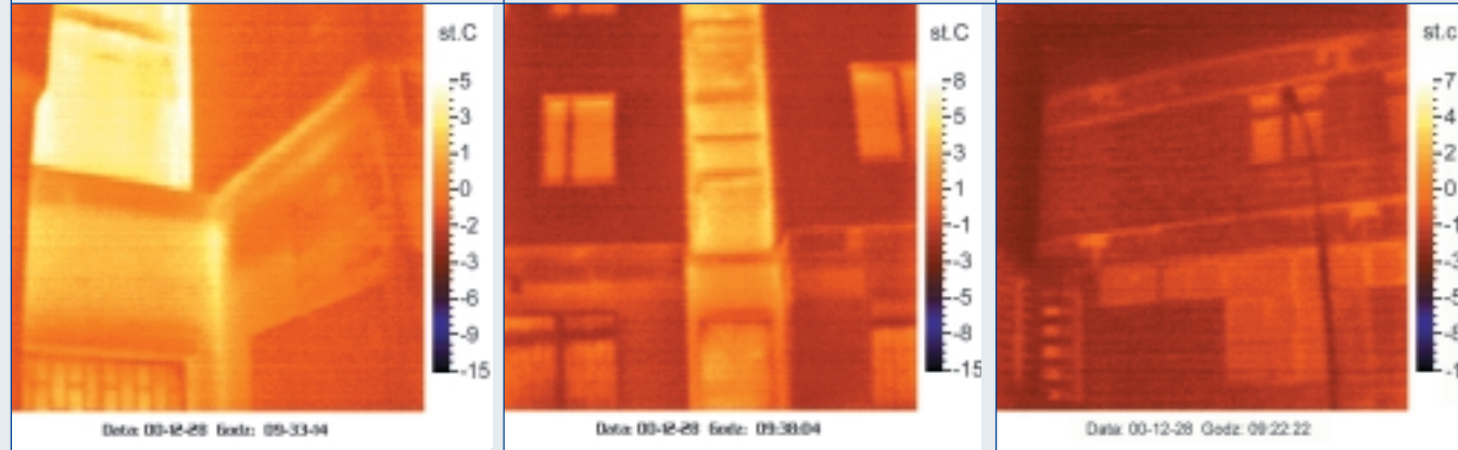
Naroże klatki schodowej budynku Klatka schodowa tego samego obiektu Ściana innego budynku (belki stropowe)
