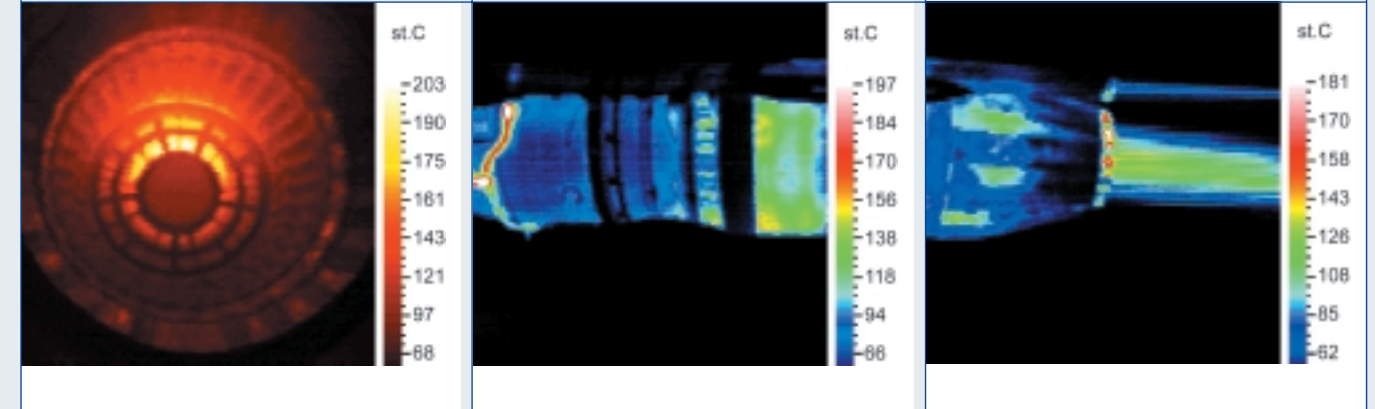
Turbina samolotu odrzutowego Poszycie silnika odrzutowego Dysza silnika odrzutowego
