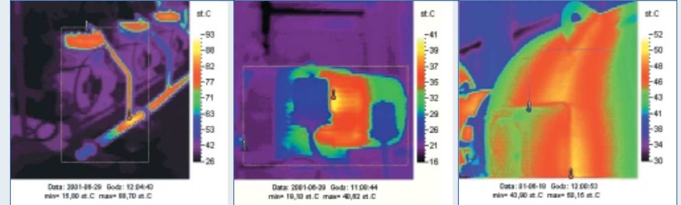
Sprężarki freonowe Silnik sprężarki amoniakalnej Korpus silnika 1250 kW
